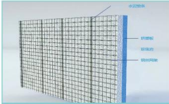
钢丝网架保温结构一体化板
